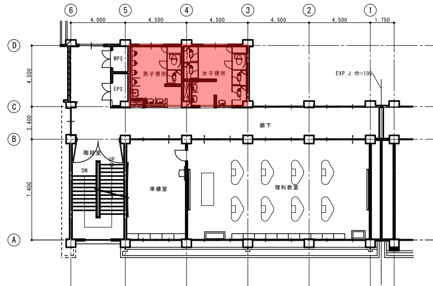
4階平面図 1/100
