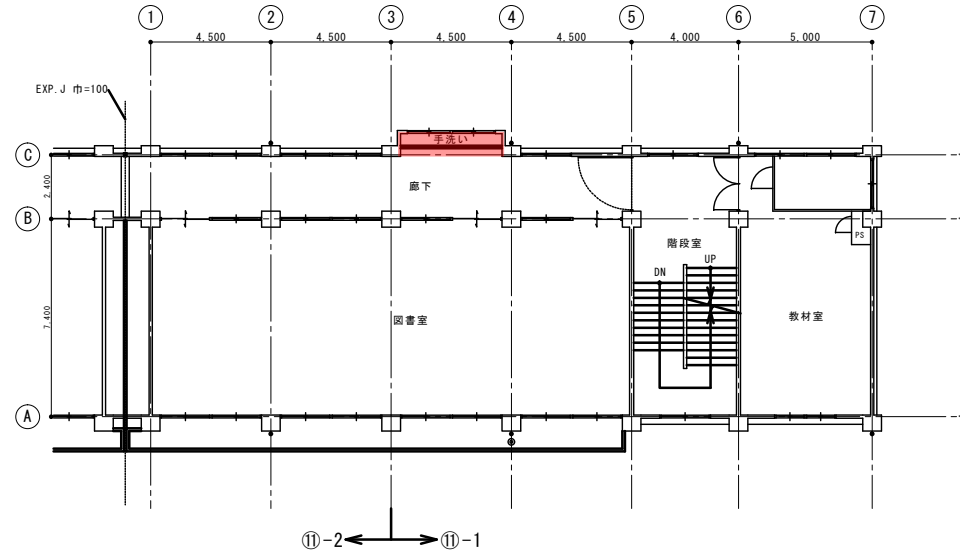
3階平面図 1/100
