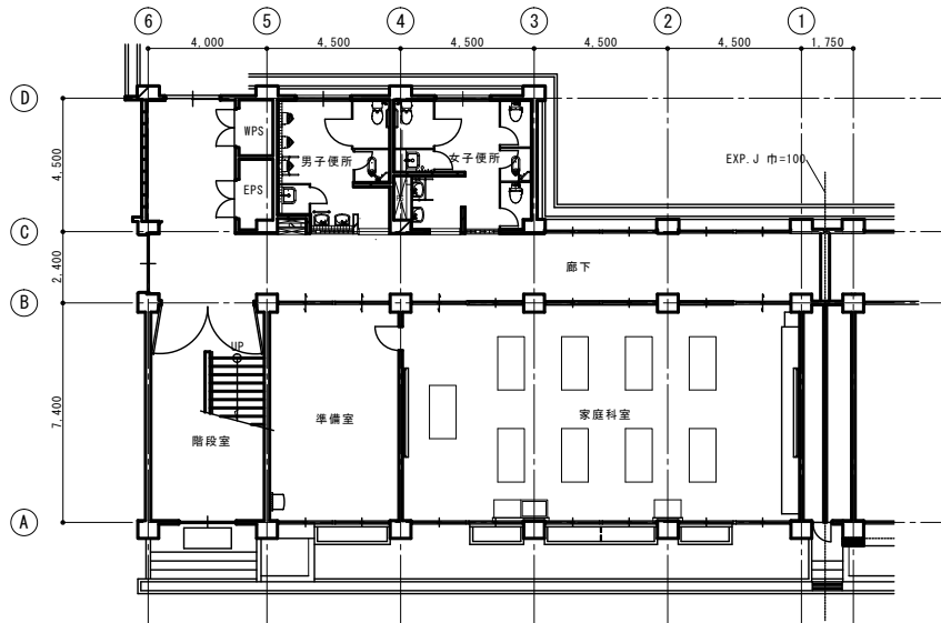
1階平面図 1/100
