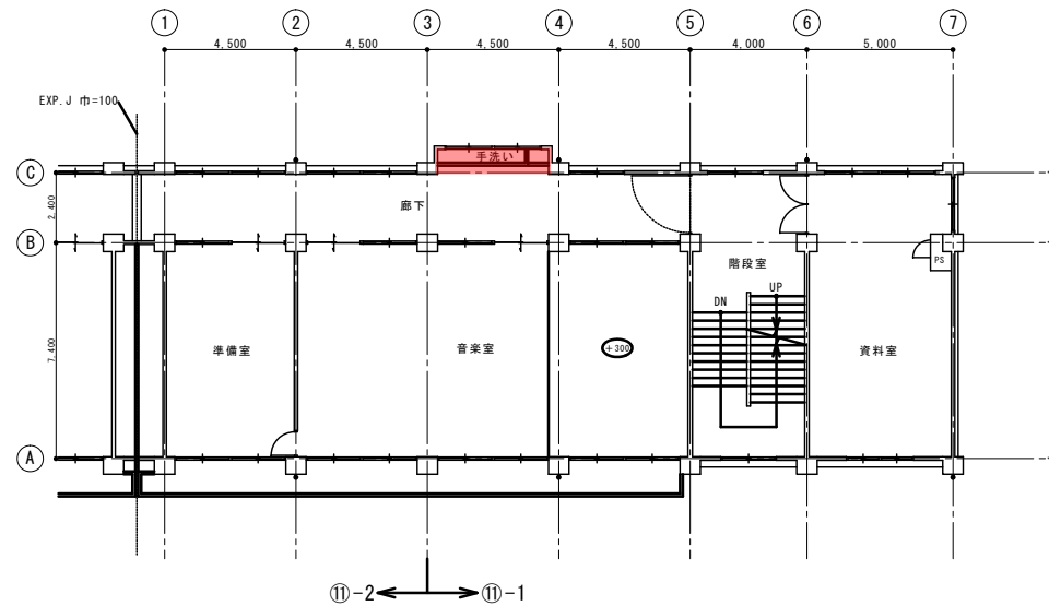
4階平面図 1/100
