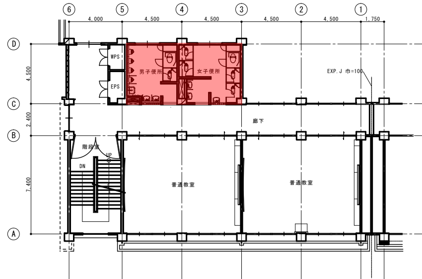
3階平面図 1/100
