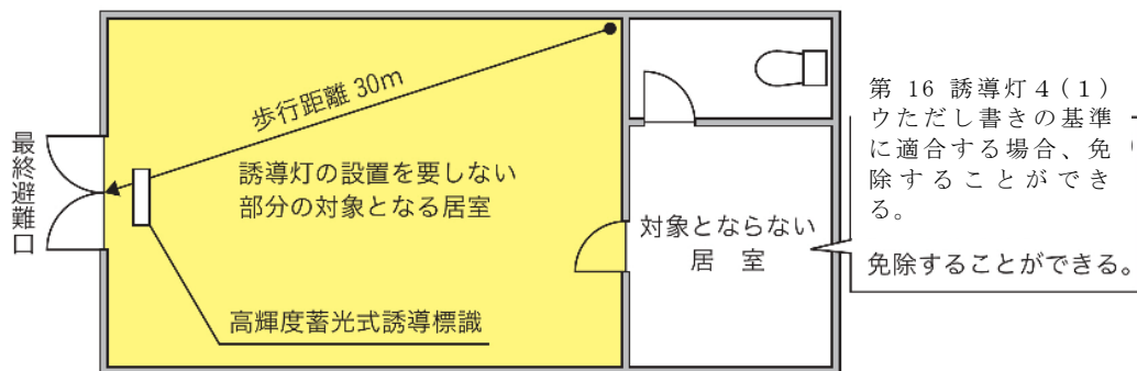
（誘導灯の設置免除の対象となる居室）
