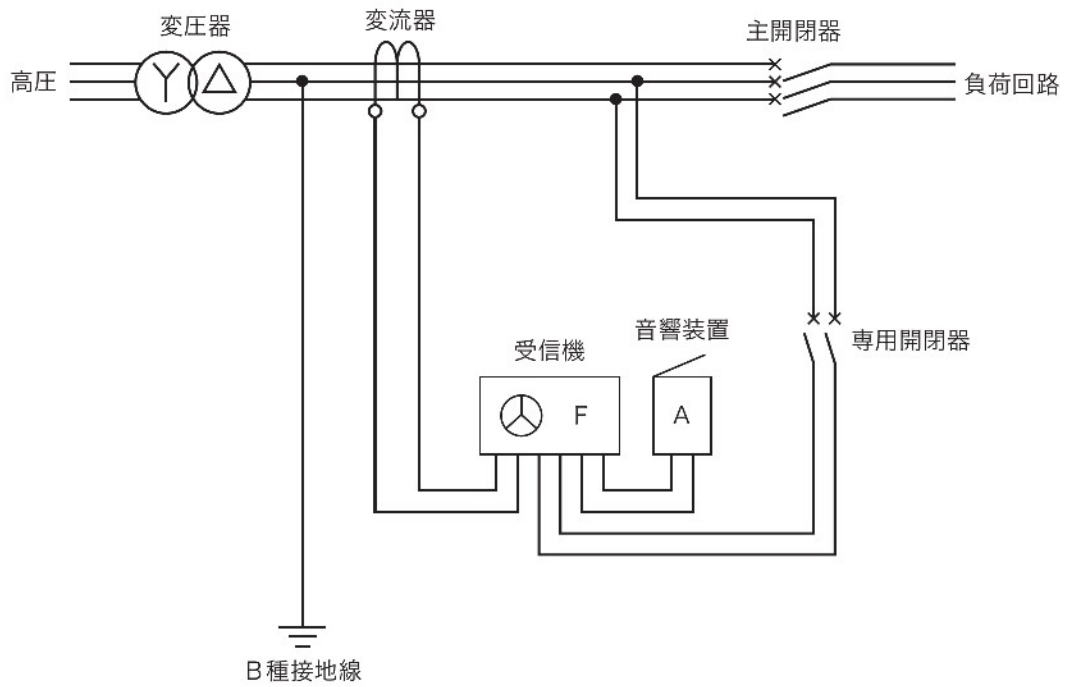
(その 3) 変圧器の二次側低圧電路に変流器を設ける方式の場合の例
