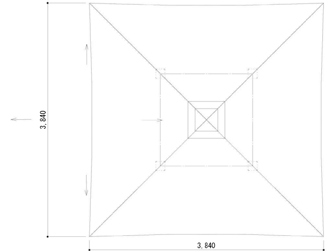
屋根伏図 1/30 0 1 2 3尺 0 0.5 1m
