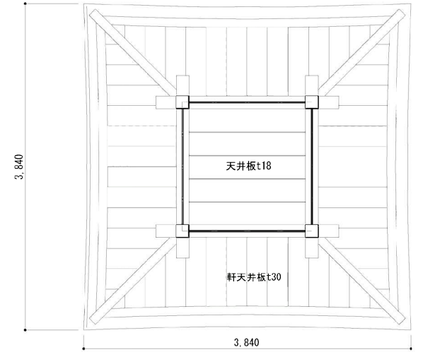
天井伏図 1:30 0 1 2 3尺 0 0.5 1m
