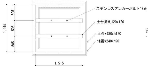
土台伏図 1:30 0 1 2 3尺 0 0.5 1m
