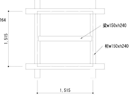
梁伏図 1:30 0 1 2 3尺 0 0.5 1m
