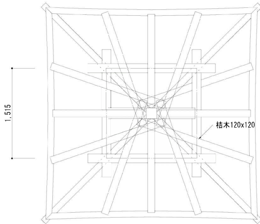
桔木伏図 1:30 0 1 2 3尺 0 0.5 1m
