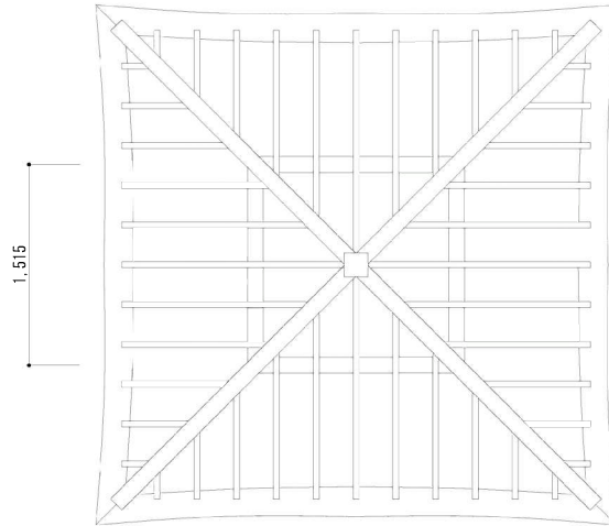
小屋伏図 1:30 0 1 2 3尺 0 0.5 1m
